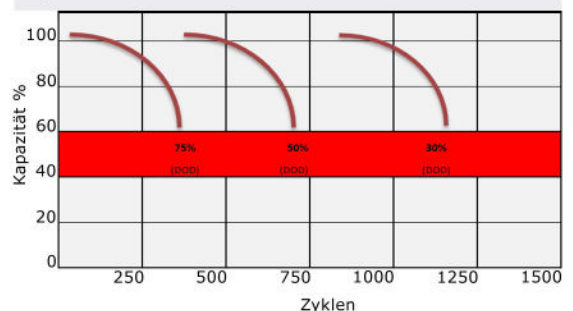
Zykluslebensdauer
