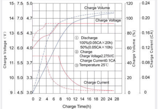
Ladecharakteristik
